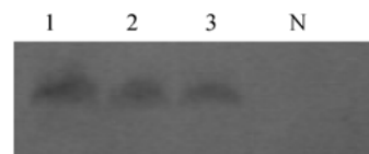
图 3 Western blot
