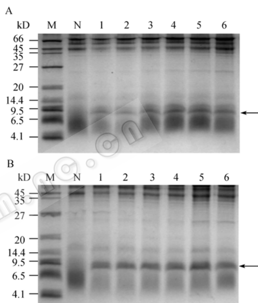
图 2 Tricine-SDS-PAGE
